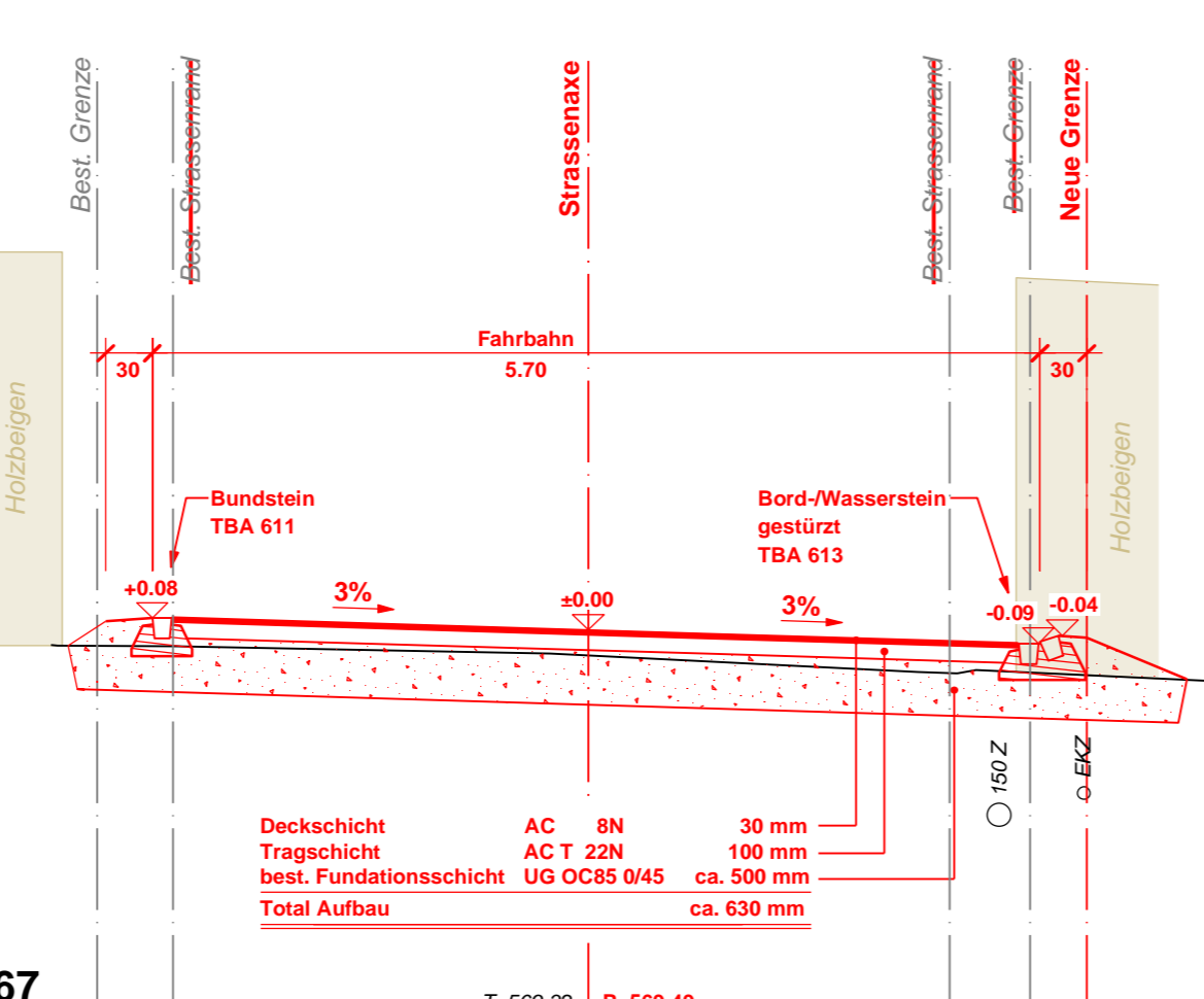
NP 1 ohne Gehweg, Km 145.00
